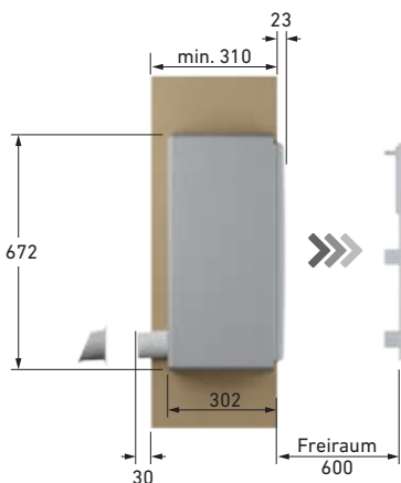
Seitenansicht SlimLine (versenkt im Wandeinbaukasten)
