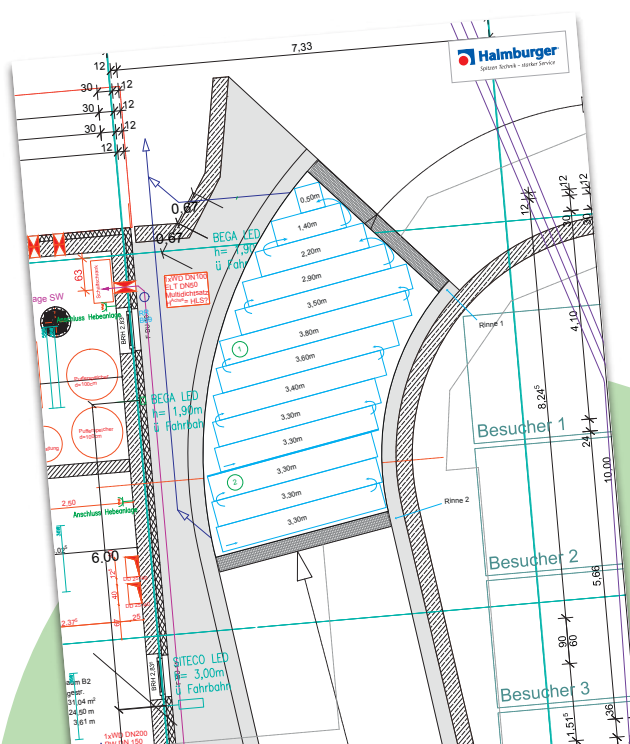
Beispiel-Skizze eines von Halmburger angefertigten Verlegeplans auf Basis eines gelieferten Grundrisses
