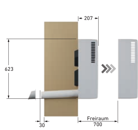
Seitenansicht Aufputz (teilversenkt)
