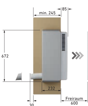
Seitenansicht Unterputz (versenkt im Wandeinbaukasten)
