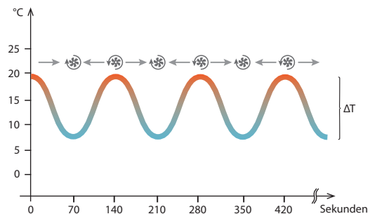
Temperaturverlauf — Richtung Luftstrom — Drehrichtung Ventilator Ⓞ
